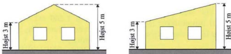
Figur 10: Maksimale højder for sommerhuse i lokalplanområdet. Skitsen stammer fra Bygningsreglement 2015 (2.2.3.3, stk. 1, nr. 2).
