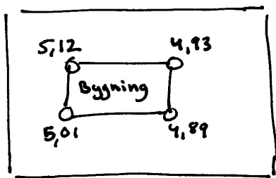
Figur 11: Niveauplanet udregnes som gennemsnittet af terrænkoterne ved bygningshjørnerne. I ovenfor illustrerede eksempel er niveauplanet derfor 4,99 = (5,12 + 5,01 + 4,93 + 4,89) / 4 .
