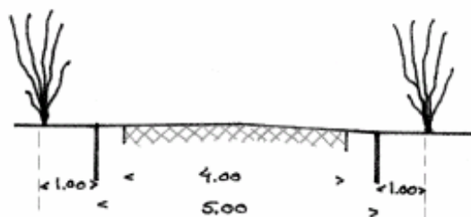
Principskitse – tværprofil af boligvej
